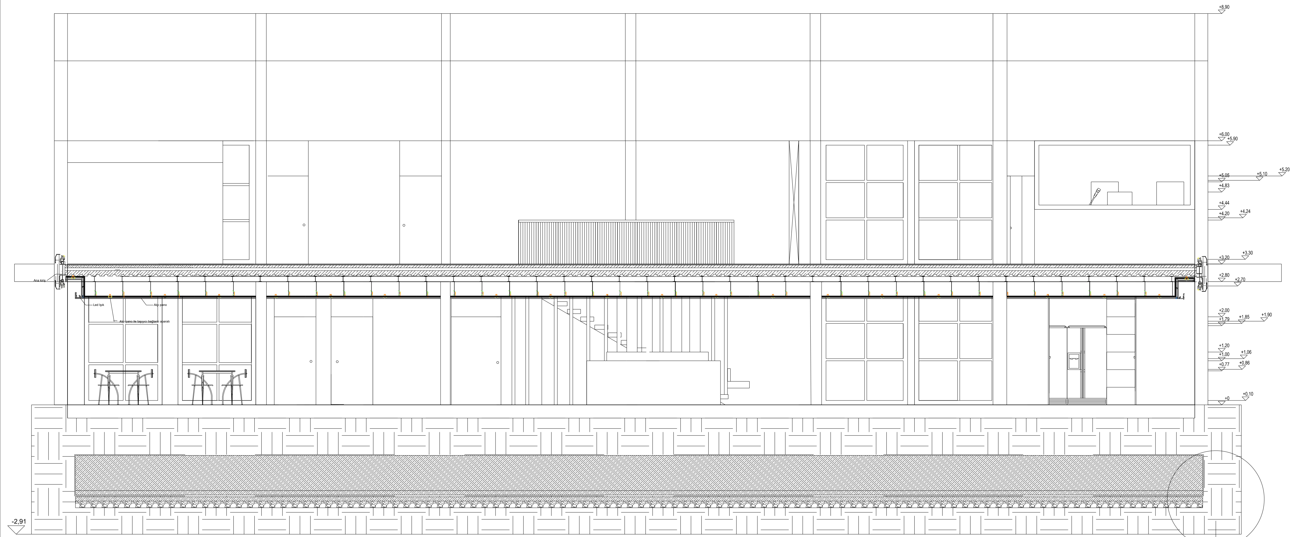
A-A1 KESİTİ 1/50
