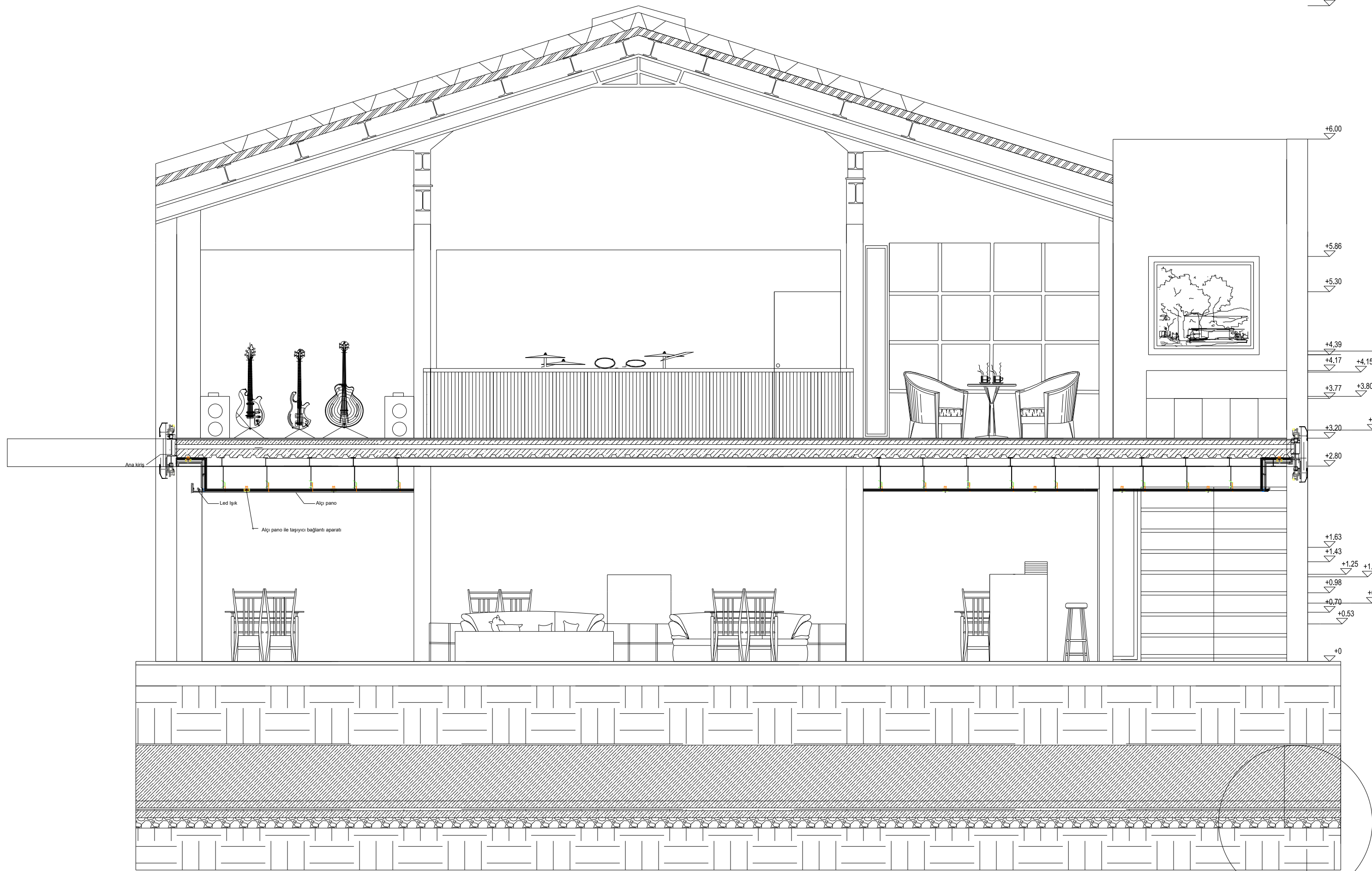
B-B1 KESİTİ 1/50
